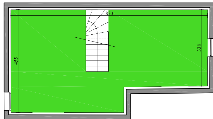
Sous-sol
